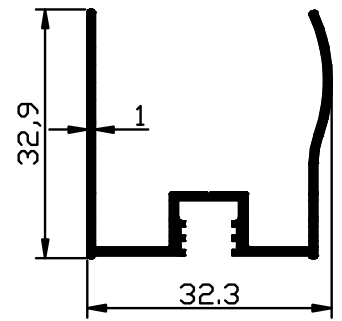
1557 - 0,313 Kg/m
