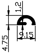
1868 - 0,052 Kg/m
