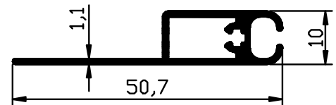
1246 - 0,305 Kg/m 600 cm
