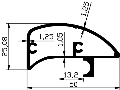
1879 - 0,569 Kg/m
