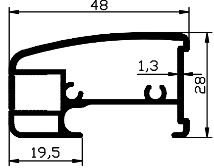
1550 - 0,710 Kg/m
