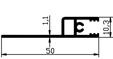
1556 - 0,289 Kg/m
