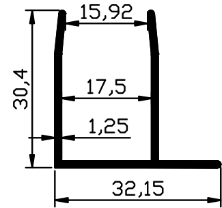
1958 - 0,305 Kg/m
