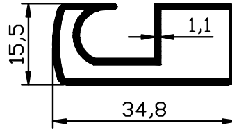
1699 - 0,356 Kg/m
