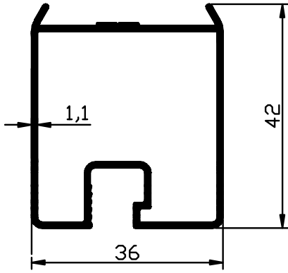
1552 - 0,537 Kg/m
