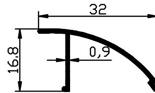
1551 - 0,146 Kg/m
