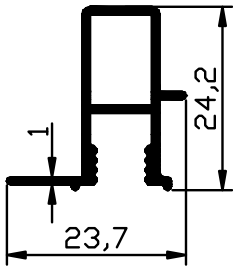
1473 - 0,235 Kg/m
