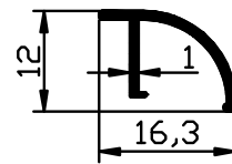
1291 - 0,089 Kg/m
