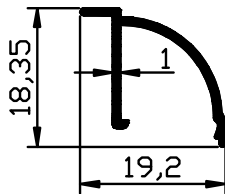
1803 - 0,122 Kg/m
