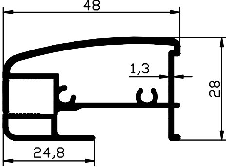
1563 - 0,716 Kg/m
