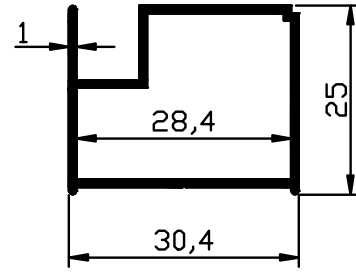
1497 - 0,314 Kg/m
