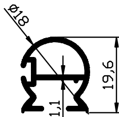
1284 - 0,240 Kg/m
