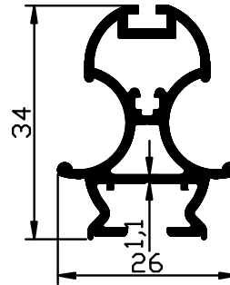
1288 - 0,448 Kg/m
