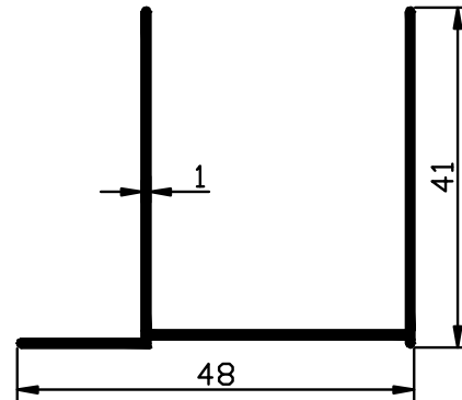
1496 - 0,345 Kg/m
