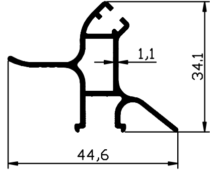
1732 - 0,365 Kg/m
