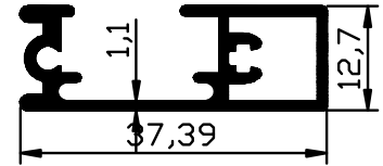
1292 - 0,359 Kg/m
