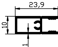
1729 - 0,226 Kg/m
