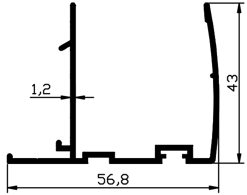
1553 - 0,532 Kg/m
