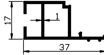
1804 - 0,276 Kg/m
