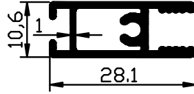
1493 - 0,297 Kg/m
