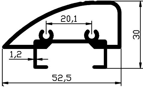
1495 - 0,734 Kg/m
