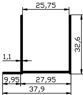
2089 - 0,300 Kg/m
