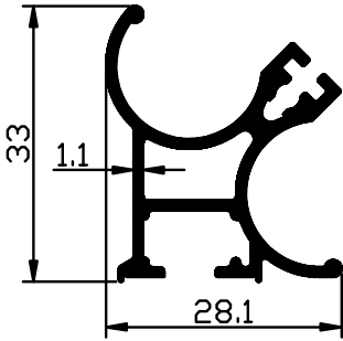
1282 - 0,540 Kg/m
