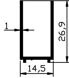
1294 - 0,179 Kg/m
