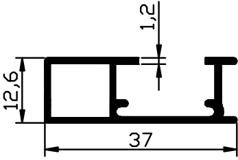
1376 - 0,296 Kg/m
