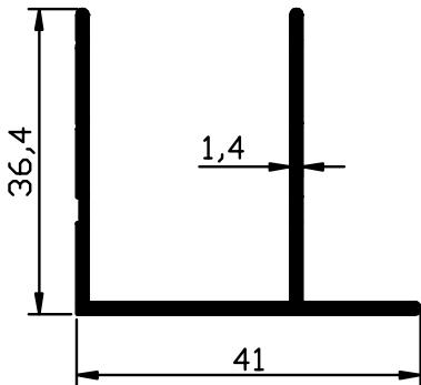
1489 - 0,418 Kg/m
