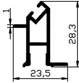
1698 - 0,278 Kg/m
