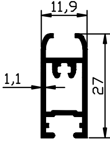
1295 - 0,279 Kg/m
