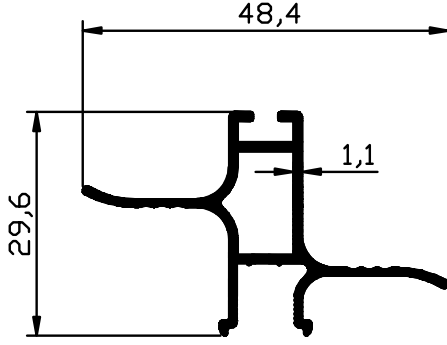
1731 - 0,355 Kg/m
