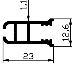
1560 - 0.205 Kg/m
