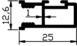
1494 - 0,237 Kg/m
