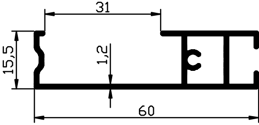
1221 - 0,463 Kg/m
