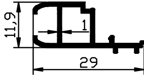
1293 - 0,203 Kg/m
