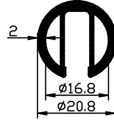
1491 - 0,401 Kg/m
