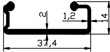
1220 - 0,335 Kg/m
