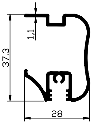
1554 - 0,400 Kg/m
