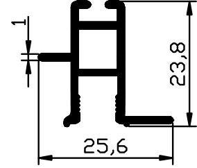
1697 - 0,273 Kg/m
