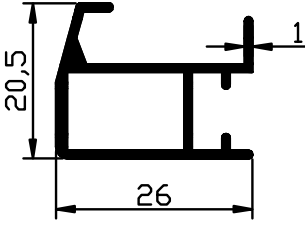
1238 - 0,286 Kg/m 600 cm
