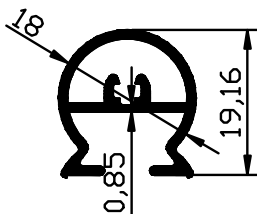
1283 - 0,243 Kg/m
