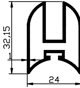
1490 - 0,416 Kg/m
