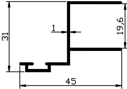
1492 - 0,282 Kg/m
