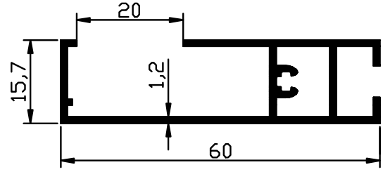
1287 - 0,508 Kg/m
