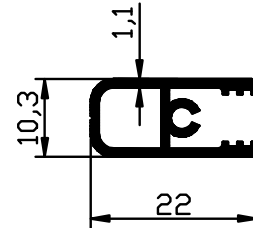
1559 - 0.209 Kg/m
