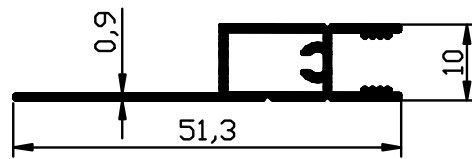
1472 - 0,273 Kg/m
