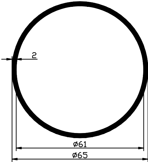
2081 1.073 Kg/m
