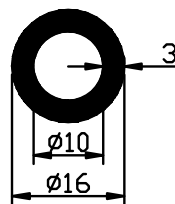
2392 2.886 Kg/m
