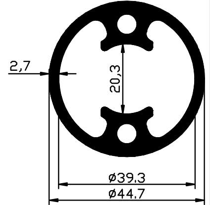
2183 1.539 Kg/m
