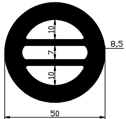
2272 3.535 Kg/m
