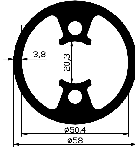
2182 - 2.778 Kg/m
