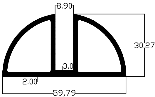
2264 - 1.068 Kg/m
