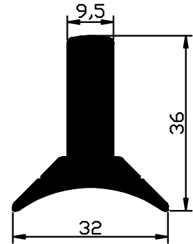
2177 1.862 Kg/m
