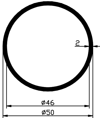
1007 - 0.813 Kg/m
