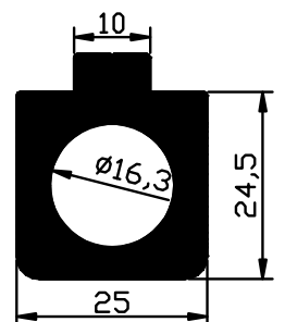
2197 1.220 Kg/m
