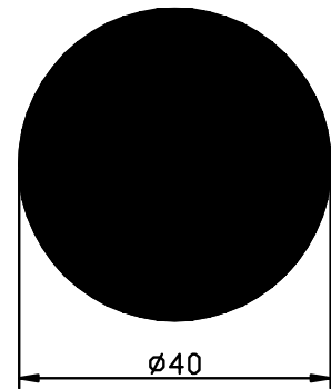
2177 1.862 Kg/m
