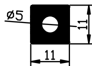
2203 0.274 Kg/m
