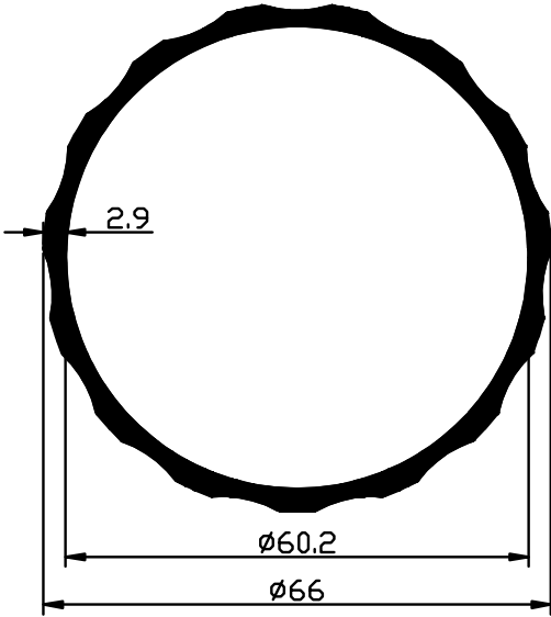
2176 - 1.313 Kg/m
