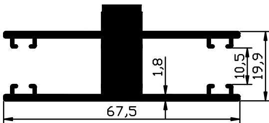
2185 1.472 Kg/m
