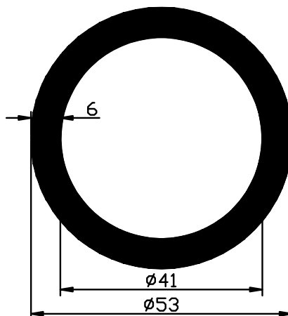
2194 2.401 Kg/m
