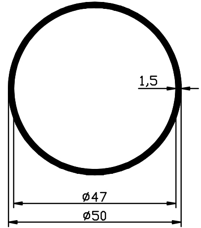
1019 - 0.616 Kg/m
