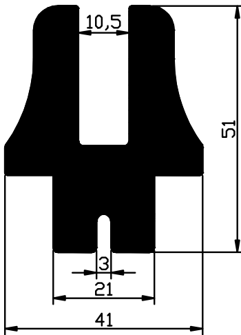
2178 4.209 Kg/m
