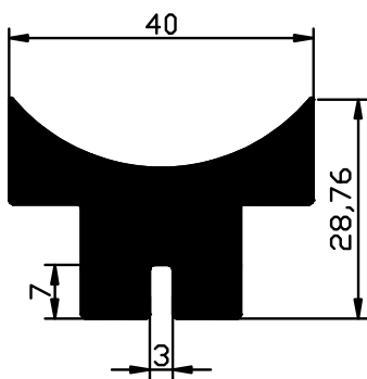
2270 1.629 Kg/m
