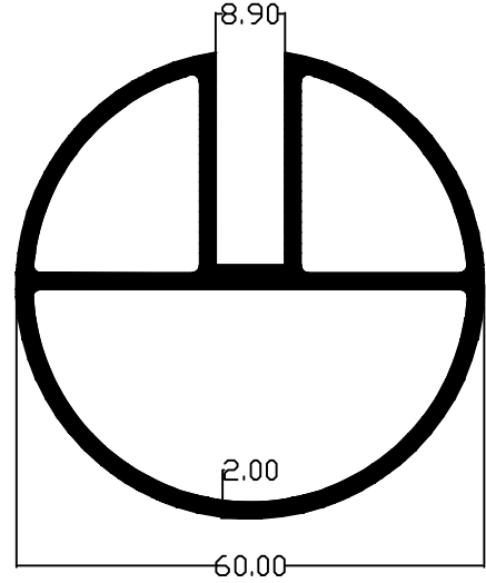
2265 1.556 Kg/m
