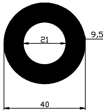
2271- 2.467 Kg/m
