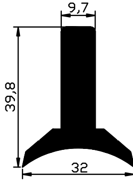
1834 - 1.187 Kg/m
