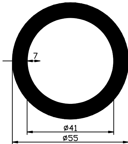
2264 - 1.068 Kg/m
