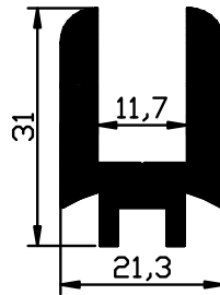
1344 - 0.867 Kg/m
