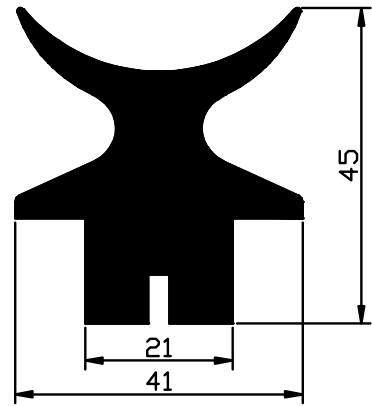
2179 2.338 Kg/m
