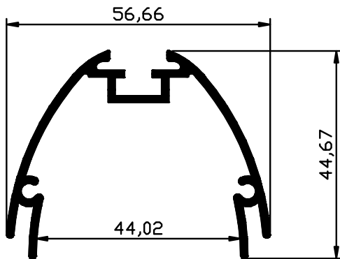
1528 - 0.706 kg/m
