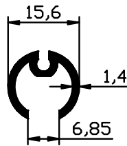
1525 - 0.168 kg/m
