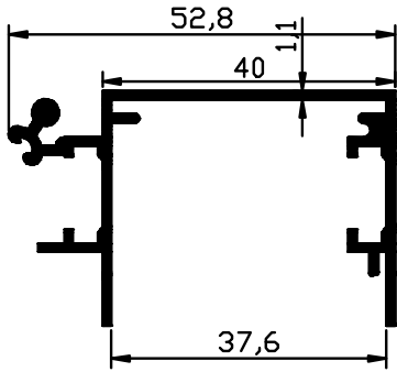
1526 - 0.551 kg/m
