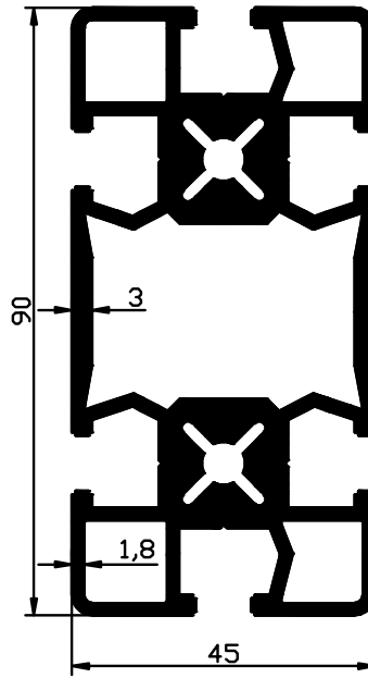
1828 - 3.450 Kg/m
