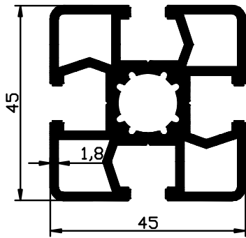
1359 - 1.670 Kg/m
