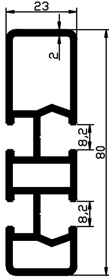
1975 1.483 Kg/m
