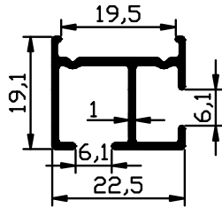
2141 - 0.228 Kg/m
