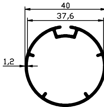
1708 - 0.468 Kg/m
