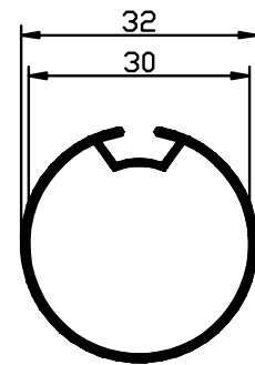
1590 - 0.284 Kg/m
