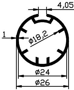
2166 - 0.282 Kg/m
