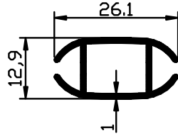
1875 - 0.212 Kg/m
