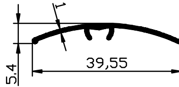
1741 - 0.137 Kg/m
