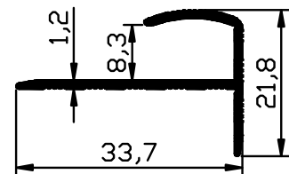
2249 - 0.115 Kg/m
