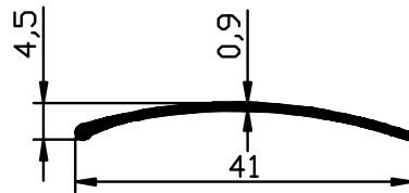
1741 - 0.137 Kg/m
