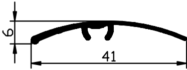
1278 - 0.149 Kg/m
