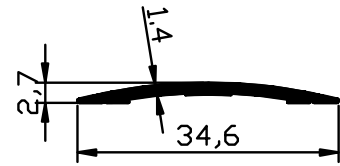
1201 - 0.145 Kg/m
