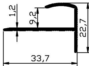
2149 - 0.203 Kg/m
