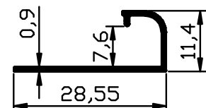
2148 - 0.115 Kg/m
