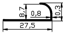
1398 - 0.089 Kg/m
