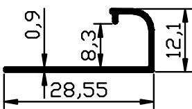
2248 - 0.115 Kg/m
