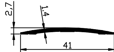
1743 - 0.127 Kg/m
