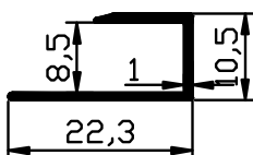
1744 - 0.110 Kg/m
