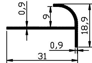
2147 - 0.131 Kg/m
