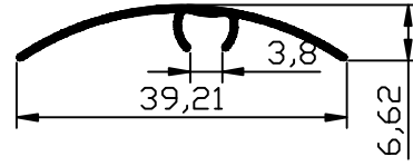
2350 - 0.114 Kg/m
