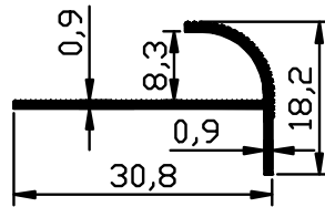
2247 - 0.115 Kg/m
