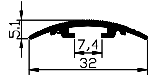
1201 - 0.145 Kg/m
