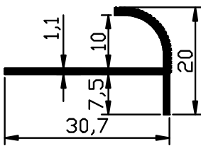
1998 - 0.174 Kg/m
