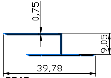
2312 - 0.123 Kg/m
