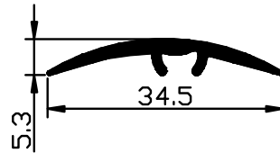
1801 - 0.176 Kg/m
