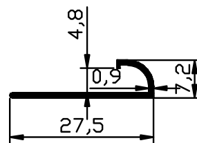
1736 - 0.092 Kg/m
